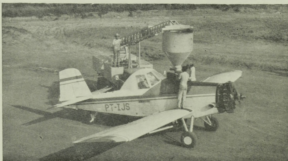
Aeronave Agrícola "THRUSH COMMANDER" de Aval, preparando-se para a aplicação de adubo granulado
