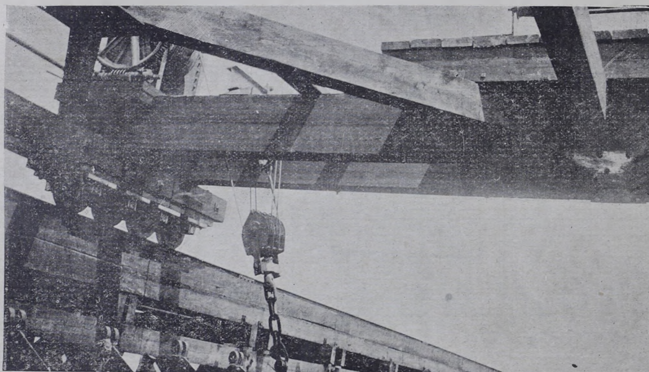
O aparelho para a construcção dos alicerces
