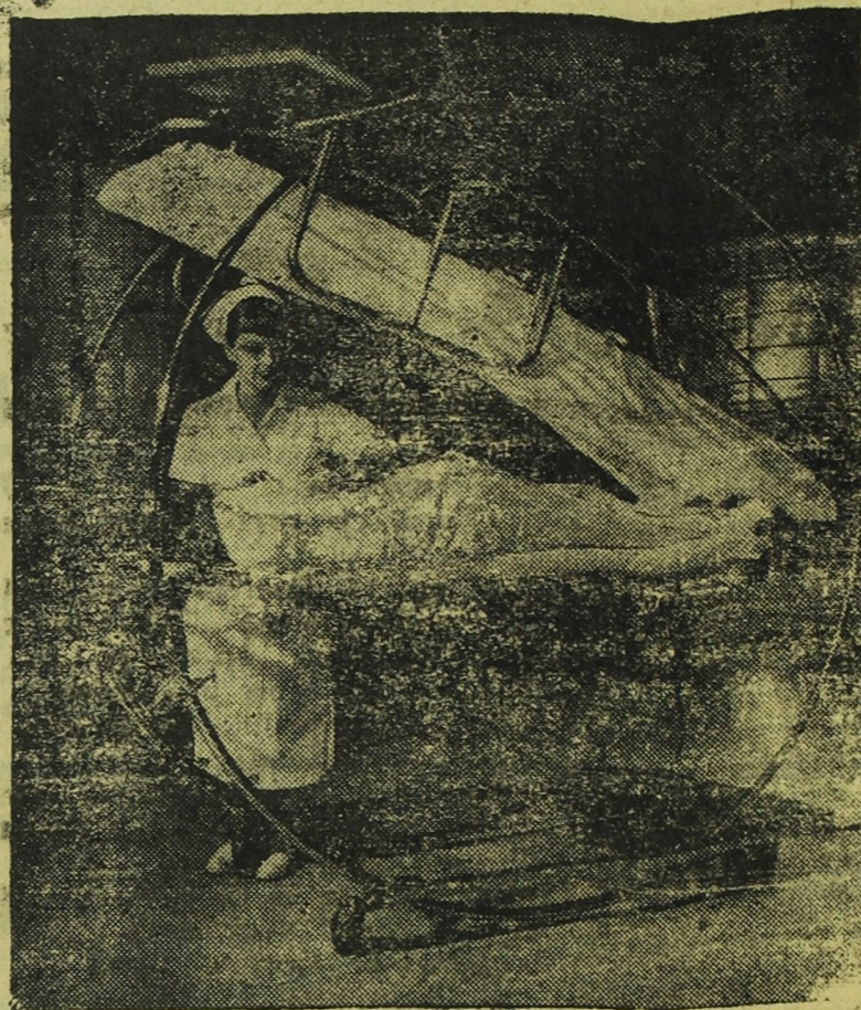
Cama de Hospital, Elétrica construída nos Estados Unidos
