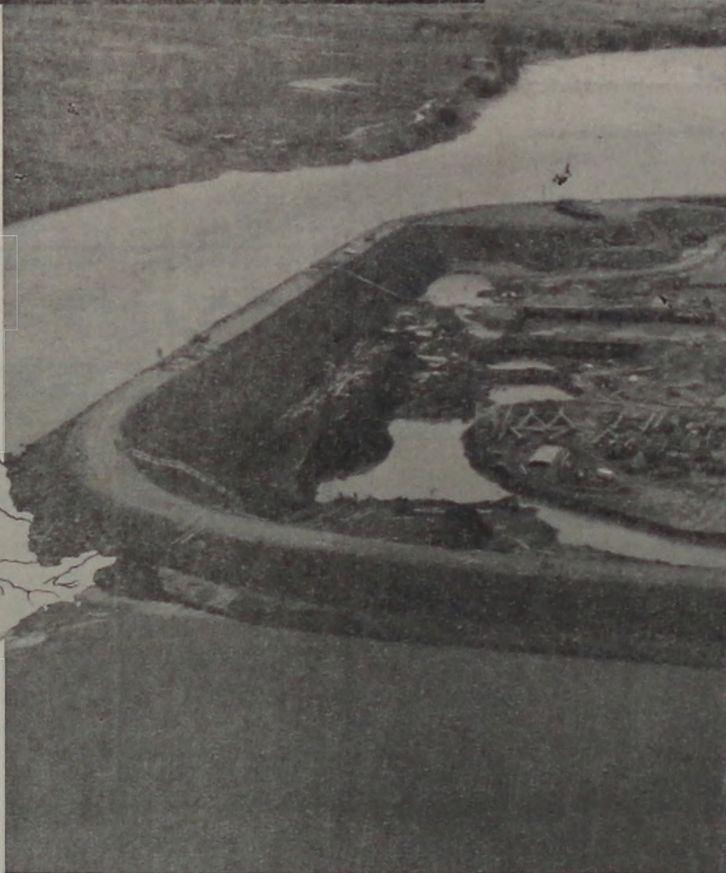
Obras da ensecadeira da Usina Nova Avanhandava, cuja primeira unidade entrará em operação em novembro de 1982.
