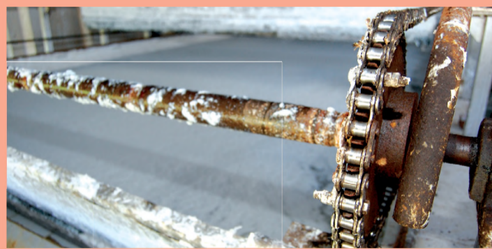
Tanque de decantação, onde ocorre a separação da água e do papel
