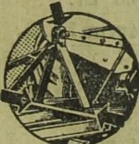
Arado de discos Dearborn, montado como parte integrante do trator Ford — não de arrasto. Com 2 discos, faz o serviço de 3.
